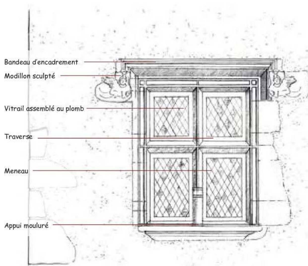
Bielle. Croisée « Renaissance ». A gauche, l'enduit couvre partiellement les pierres qui composent l'encadrement afin de souligner la régularité et la qualité de cet élément architectural. Les parties irrégulières ne sont pas laissées à la vue, l'encadrement est composé à la fois par la pierre sculptée et par l'enduit.
