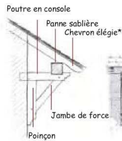
Débord de toit sur console.
